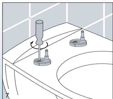
Serrer les vis
