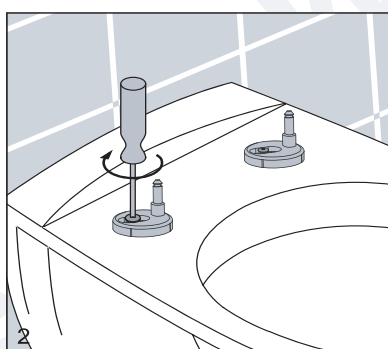
Serrer les vis des charnières
