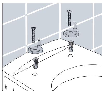
Insérer les charnières dans la toilette
