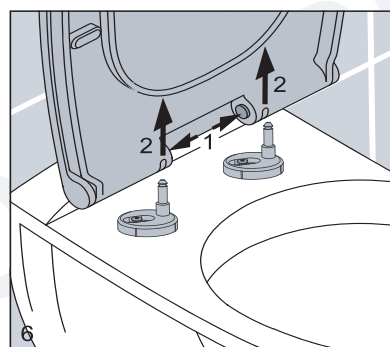
Retirer le siège et le couvercle des toilettes en appuyant sur les deux boutons-poussoirs
