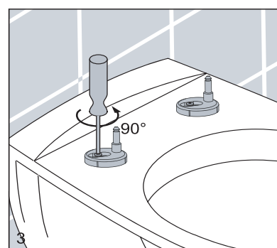
Desserrer légèrement les vis en les tournant à 90° vers la droite
