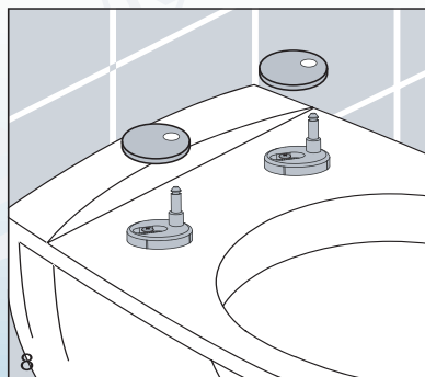
Placer les capuchons de recouvrement sur les charnières
